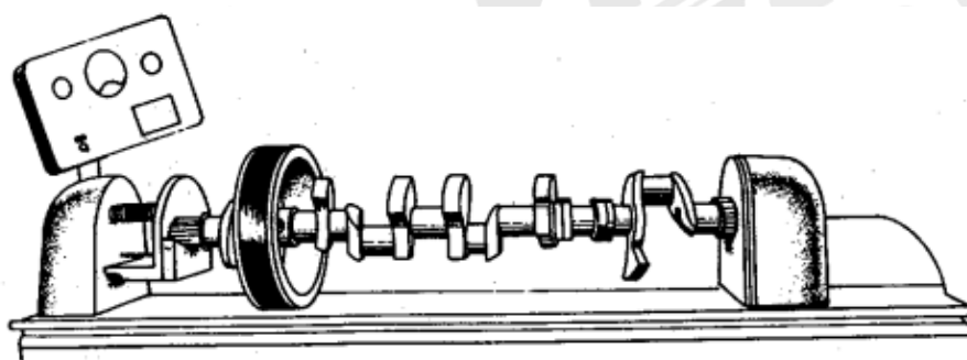
Figura 10-6 Magnetização longitudinal do eixo manivela (método do solenoide).
