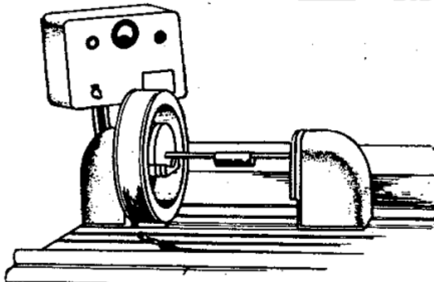
Figura 10-4 Magnetização circular de um eixo manivela.
