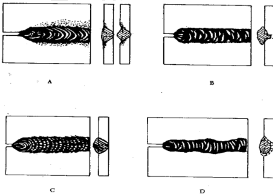
Figura 10-22 Exemplos de soldas mal feitas.
