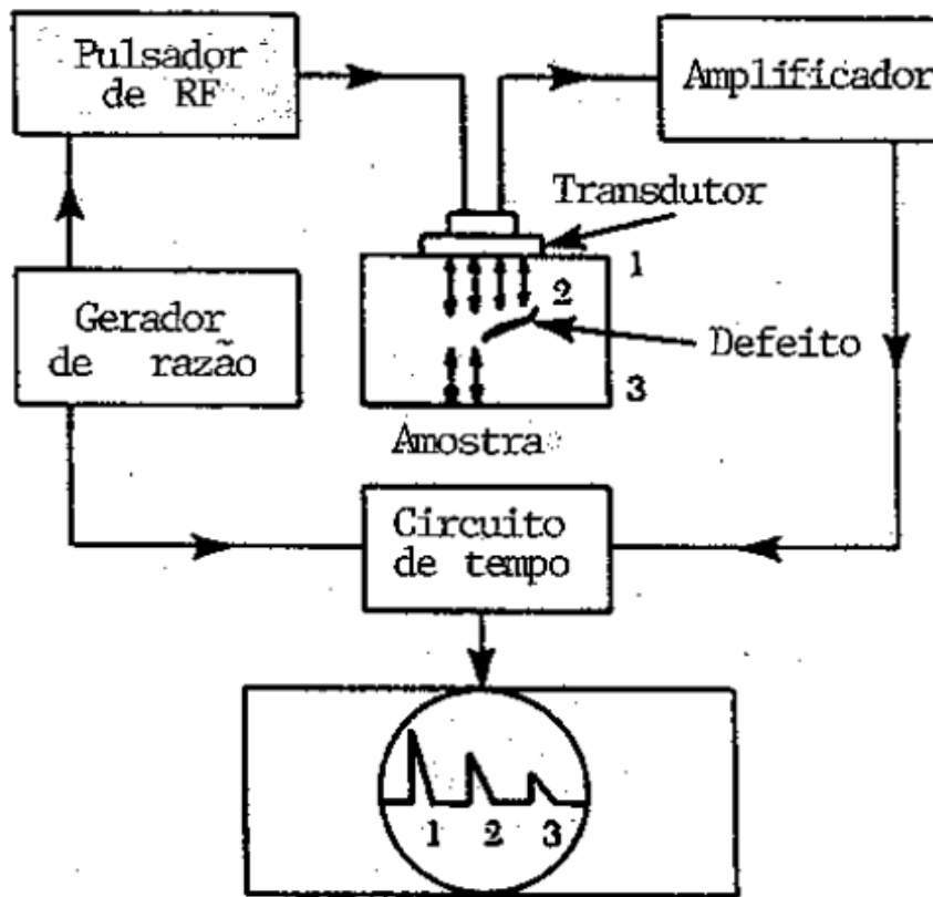
Osciloscópio de raio catodo
